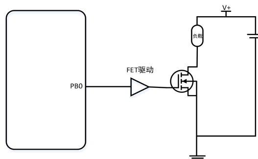
单 PWM 电路
