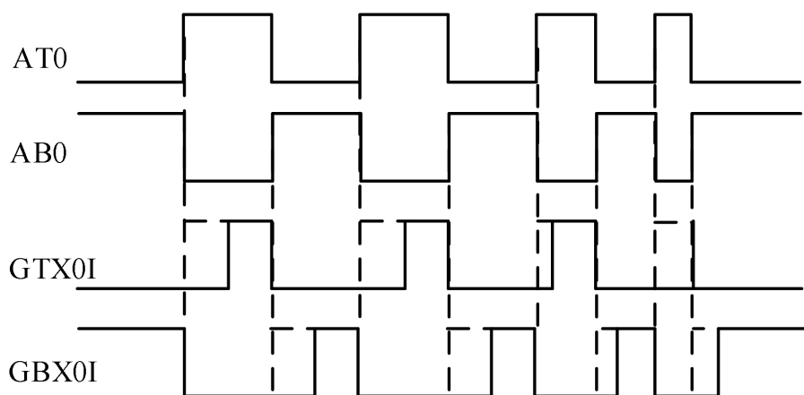
死区时间方框图
