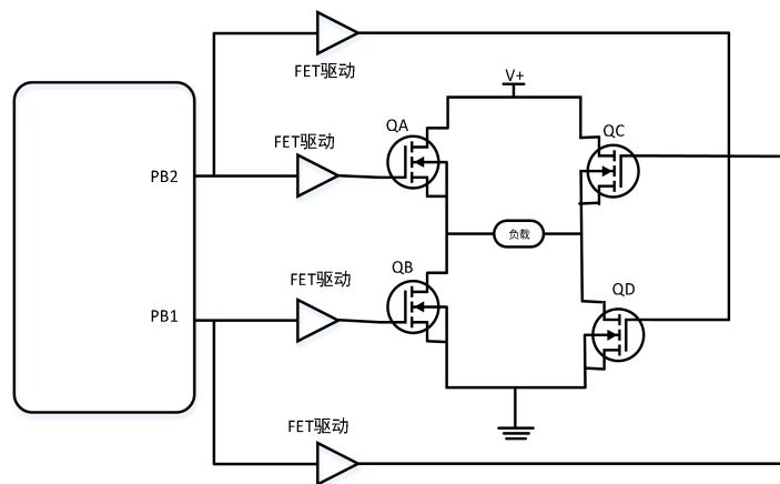
半桥输出驱动全桥电路（4NMOS）注：PB0 和 PA0, PA1 和 PA2 同图上一样
