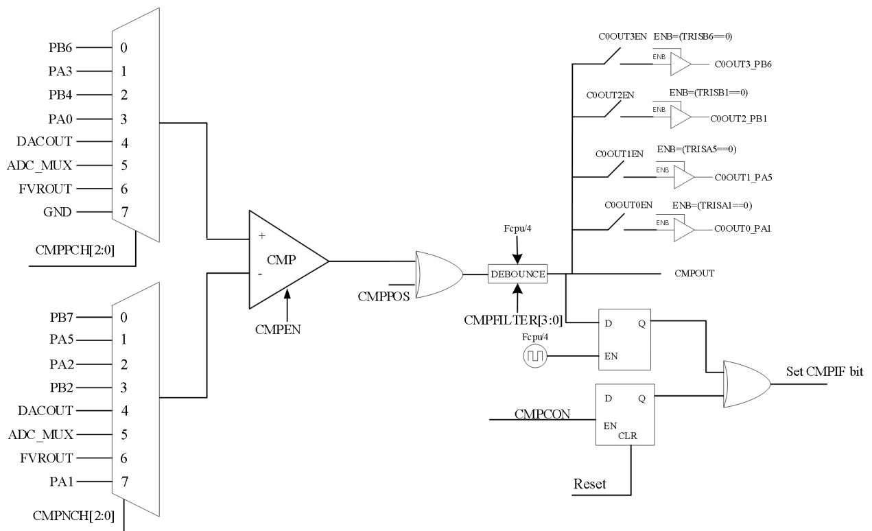
CMP 电路图
