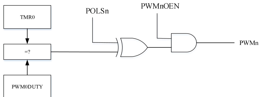
PWM 原理框图 (n=0)
