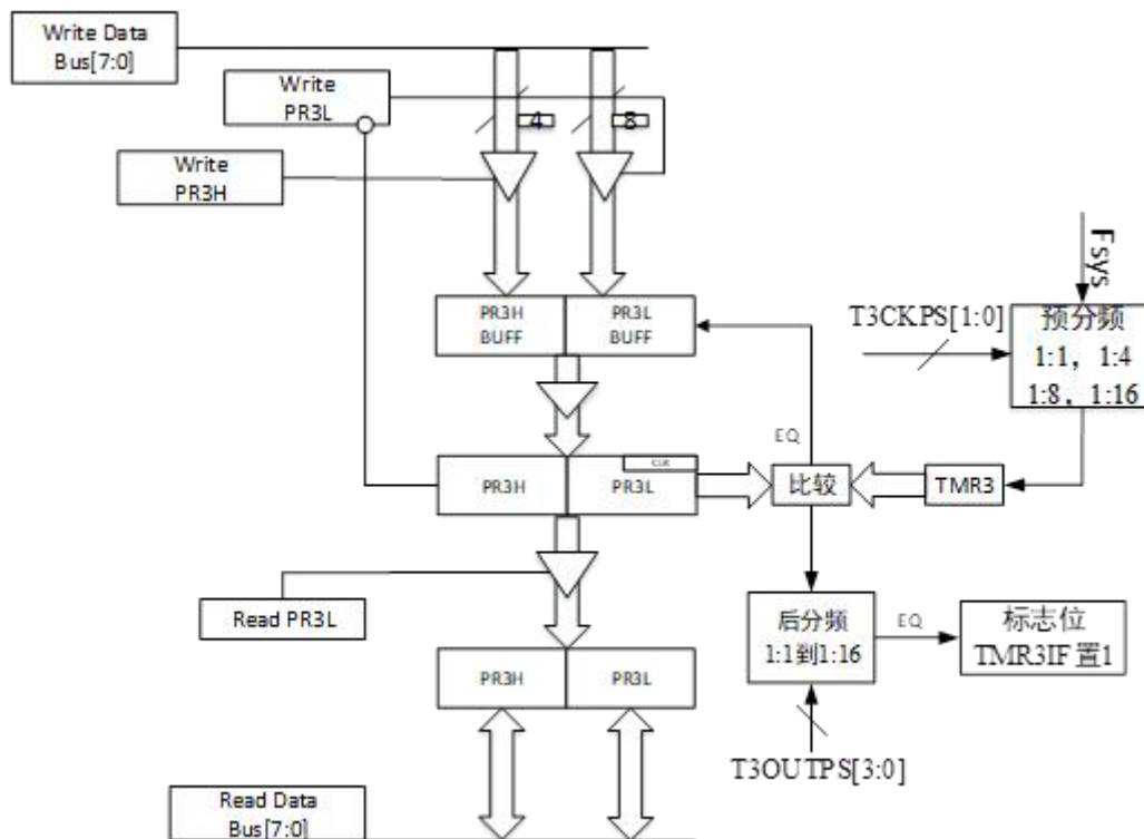
T3 结构图
