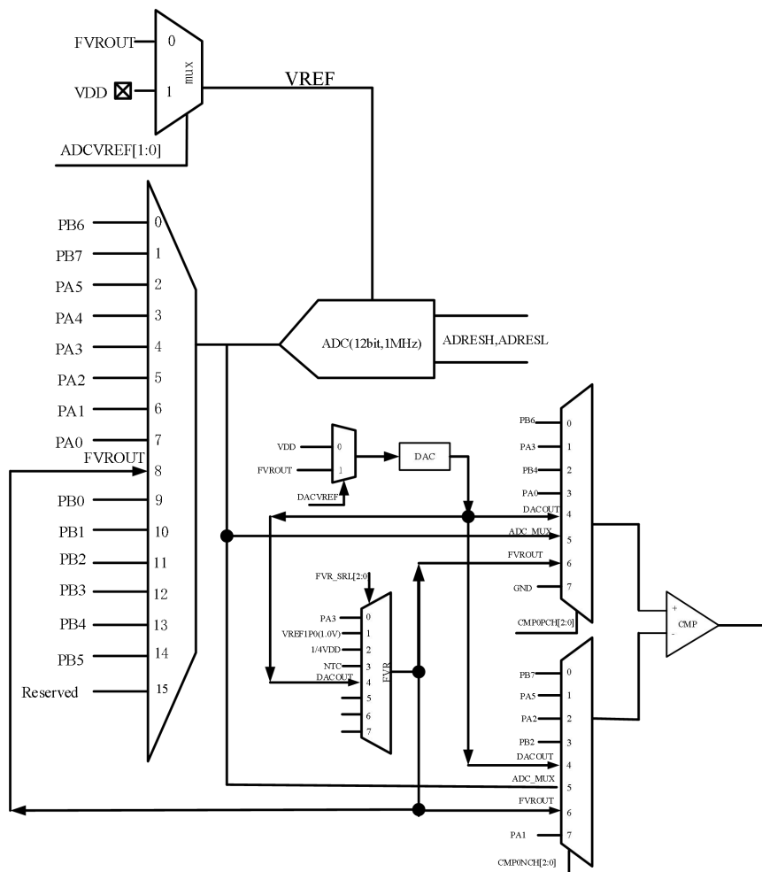
模块关系图
