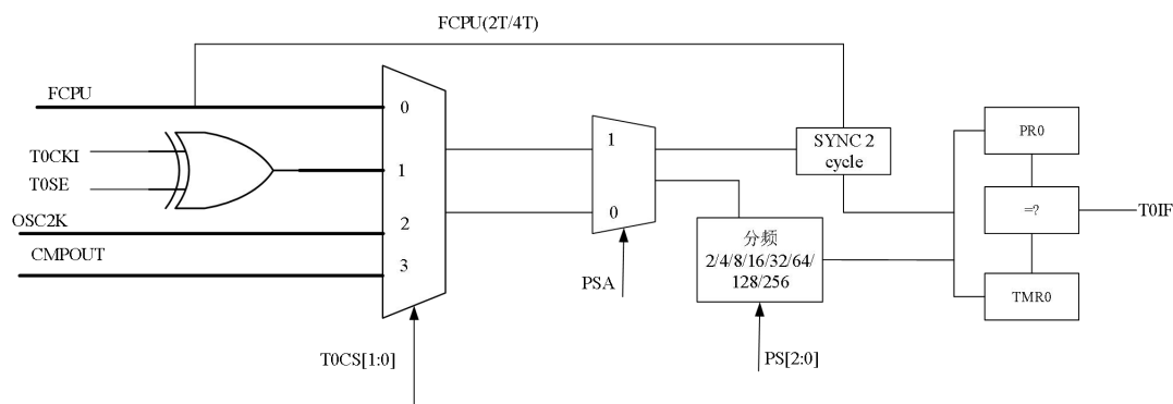
Timer0 结构图
